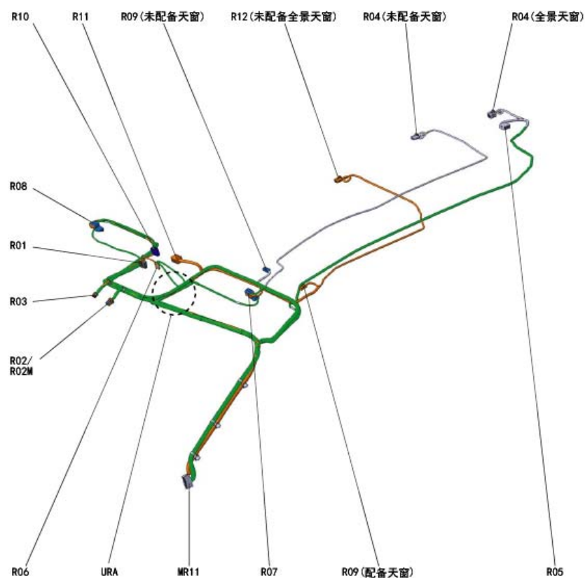
车顶线束
